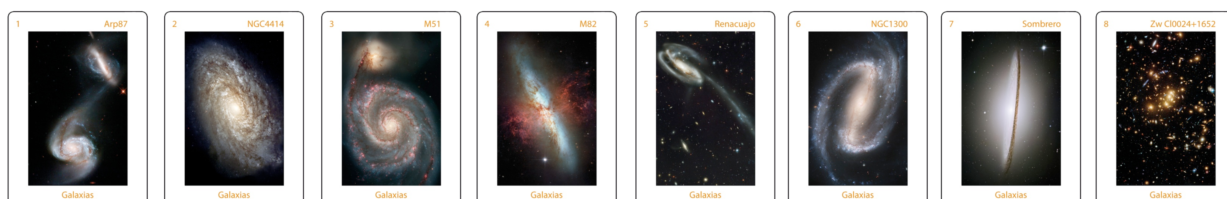
Galaxies
