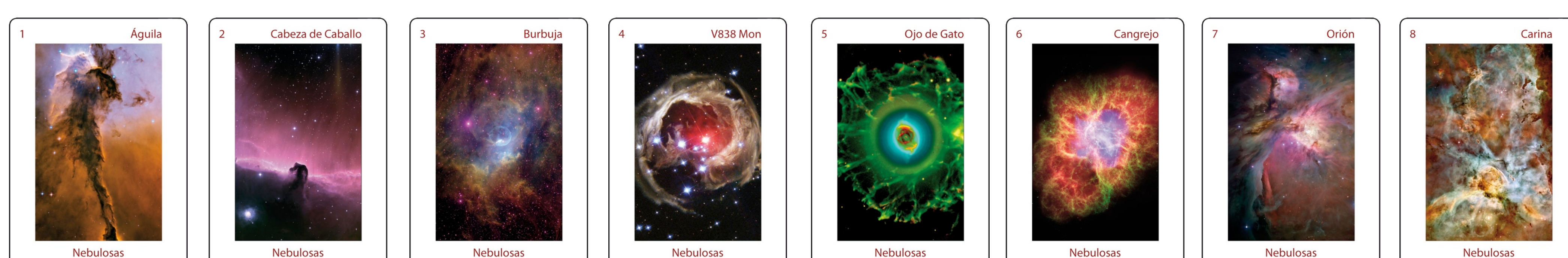
Nebulae
